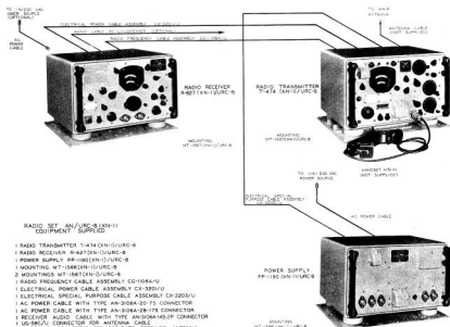
Radio Set AN/URC-8(XN-1)
